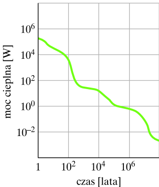
Rys. 44.6. Moc cieplna wyzwalana w czasie rozpadu odpadów promieniotwórczych nagromadzonych w czasie rocznej pracy typowej elektrowni jądrowej. Przebieg krzywej jest wynikiem nałożenia efektów związanych z rozpadem wielu nuklidów o różnych czasach połowicznego zaniku. Zwróćcie uwagę, że obydwie osie wykresu mają skalę logarytmiczną
