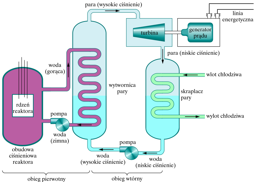
Rys. 44.5. Uproszczony schemat elektrowni jądrowej z reaktorem wodnym ciśnieniowym. Pominięto wiele szczegółów budowy — w tym układy chłodzące rdzeń reaktora w razie awarii
