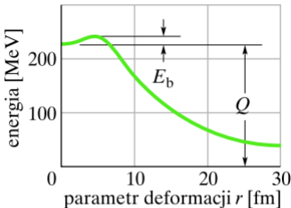
Rys. 44.3. Energia potencjalna jądra na różnych etapach reakcji rozszczepienia według przewidywań modelu Bohra i Wheelera. Na wykresie zaznaczono energię rozszczepienia Q (około 200 MeV) i wysokość bariery E_b
