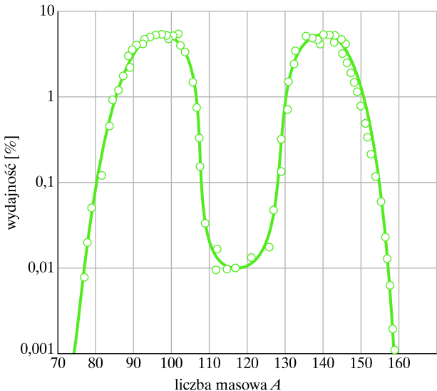
Rys. 44.1. Rozkład mas fragmentów powstałych w wyniku rozszczepienia nuklidu ^{235}\text{U} . Zwróć uwagę, że oś pionowa jest w skali logarytmicznej
