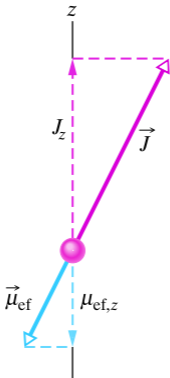
Rys. 41.7. Klasyczny model pokazujący wektor całkowitego momentu pędu \vec{J} i wektor efektywnego momentu magnetycznego \vec{\mu}_{\text{ef}}
