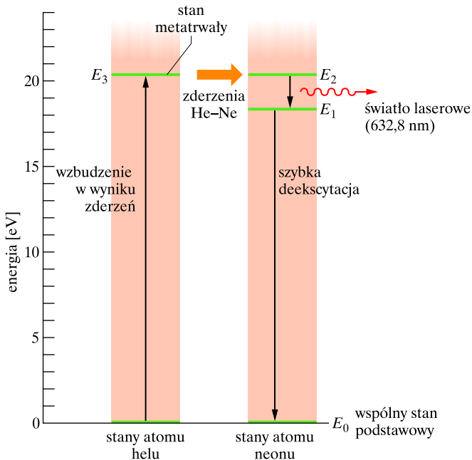
Rys. 41.22. Cztery poziomy energetyczne atomów helu i neonu, kluczowe dla działania lasera helowo-neonowego. Akcja laserowa zachodzi pomiędzy poziomami neonu E_2 i E_1 , gdy na poziomie E_2 znajduje się więcej atomów niż na poziomie E_1
