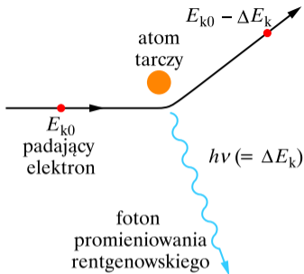
Rys. 41.15. Elektron o energii kinetycznej E_{k0} przelatujący obok atomu w tarczy może wyemitować foton promieniowania rentgenowskiego, tracąc przy tym część swojej energii. W taki sposób powstaje widmo ciągłe promieniowania rentgenowskiego
