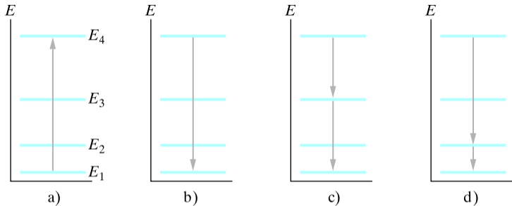
Rys. 40.4. a) Wzbudzenie uwięzionego elektronu ze stanu podstawowego do trzeciego stanu wzbudzonego. b)–d) Trzy z czterech możliwych sposobów powrotu elektronu ze stanu wzbudzonego do stanu podstawowego. (Jaki sposób nie został pokazany?)
