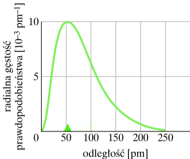
Rys. 40.18. Rozkład radialnej gęstości prawdopodobieństwa P(r) dla stanu podstawowego atomu wodoru. Trójkąt został umieszczony w odległości jednego promienia Bohra od początku układu współrzędnych. Początek układu współrzędnych oznacza środek atomu
