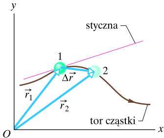
Rys. 4.4. Przemieszczenie \Delta\vec{r} cząstki w przedziale czasu \Delta t . W chwili początkowej t_1 cząstka znajduje się w punkcie 1, o wektorze położenia \vec{r}_1 , a w chwili końcowej t_2 — w punkcie 2, o wektorze położenia \vec{r}_2 . Pokazano styczną do toru cząstki w punkcie 1
