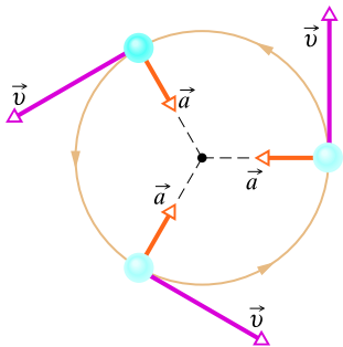
Rys. 4.18. Wektory przyspieszenia i prędkości cząstki poruszającej się jednostajnie po okręgu, w kierunku przeciwnym do kierunku ruchu wskazówek zegara. Obydwa mają stałą długość, lecz ich kierunki zmieniają się w sposób ciągły
