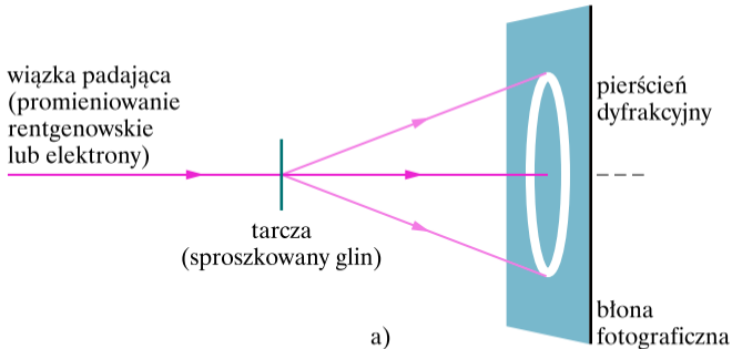
Rys. 39.9. a) Układ doświadczalny wykorzystywany do prezentacji falowego charakteru padającej wiązki metodami dyfrakcyjnymi.
