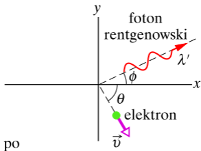
Rys. 39.5. Foton promieniowania rentgenowskiego o długości fali \lambda oddziałuje z nieruchomym elektronem. Zostaje on rozproszony pod kątem \phi i jego długość fali \lambda' się zwiększyła. Elektron porusza się po zderzeniu z prędkością v pod kątem \theta
