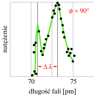
Rys. 39.4. Wyniki doświadczenia Comptona dla czterech wartości kąta rozpraszania \phi . Zauważ, że przesunięcie comptonowskie \Delta\lambda zwiększa się wraz ze wzrostem kąta rozpraszania
