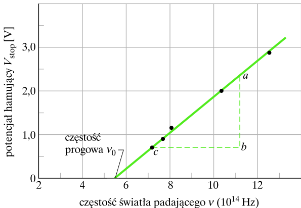
Rys. 39.2. Zależność potencjału hamującego V_{\text{stop}} od częstości \nu światła padającego na elektrodę wykonaną z sodu w układzie doświadczalnym z rysunku 39.1 (dane opublikowane przez R.A. Millikana w 1916 r.)
