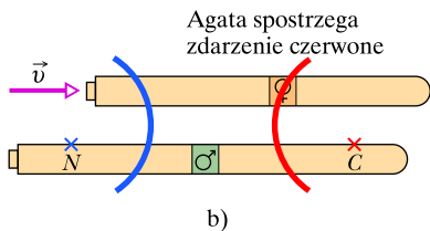
Rys. 38.4. Statki kosmiczne Agaty i Jacka oraz zdarzenia narysowane tak, jak widzi je Jacek. Statek Agaty porusza się w prawo z prędkością \vec{v} . a) Zdarzenie czerwone zachodzi w punktach C i C' , a zdarzenie niebieskie w punktach N i N' ; obydwa zdarzenia są źródłem fali świetlnej. b) Agata spostrzega czoło fali od zdarzenia czerwonego. c) Jacek jednocześnie spostrzega czoła fal od zdarzenia czerwonego i zdarzenia niebieskiego. d) Agata spostrzega czoło fali od zdarzenia niebieskiego.
