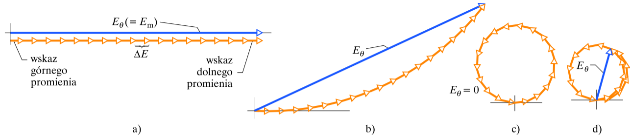
Rys. 37.6. Diagramy dla N = 18 wskaźów odpowiadających podziałowi pojedynczej szczeliny na 18 stref. Pokazane na rysunkach wypadkowe amplitudy E_\theta odnoszą się do: a) centralnego maksimum ( \theta = 0 ), b) punktu na ekranie, którego położenie jest bliskie osi (mały kąt \theta ), c) pierwszego minimum oraz d) pierwszego maksimum bocznego
