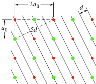
Rys. 37.27. Rodzina płaszczyzn odbijających (płaszczyzn sieciowych) w strukturze kryształu z rysunku 37.26a i objaśnienie, jak długość krawędzi komórki elementarnej a_0 wiąże się z odległością międzypłaszczyznową d
