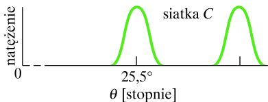
Rys. 37.24. Krzywe natężenia dla światła o dwóch długościach fali, przechodzącego przez siatki dyfrakcyjne wymienione w tabeli 37.1. Siatka B ma największą zdolność rozdzielczą, a siatka C największą dyspersję
