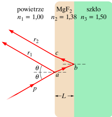
Rys. 36.15. Przykład 36.5. Niepożądane odbicia od szkła można wyeliminować (dla wybranych długości fali), pokrywając szkło cienką przezroczystą warstwą fluorku magnezu o odpowiednio dobranej grubości
