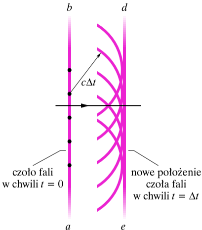
Rys. 36.1. Konstrukcja geometryczna Huygensa ilustrująca rozchodzenie się fali płaskiej w próżni
