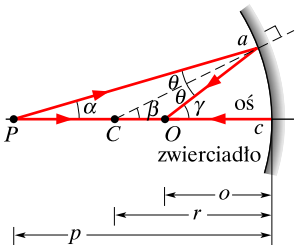
Rys. 35.19. Sferyczne zwierciadło wklęsłe, odbijając promienie świetlne przychodzące z punkowego przedmiotu, wytwarza rzeczywisty obraz punktowy O tego przedmiotu
