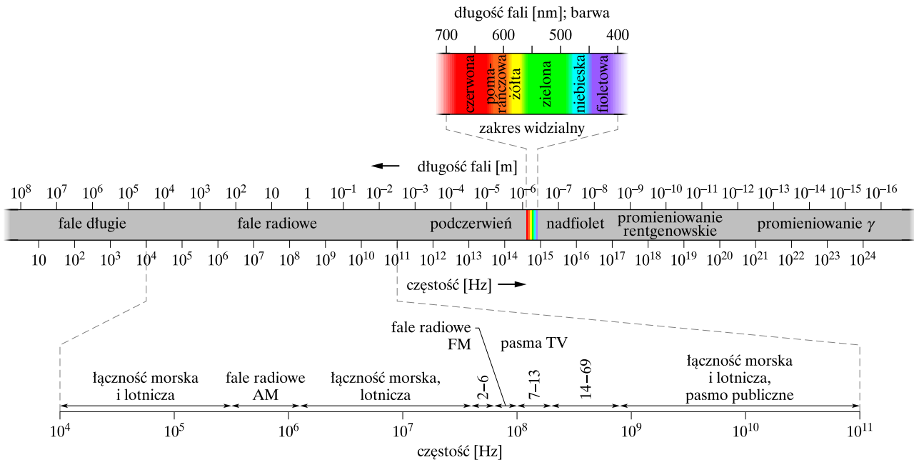
Rys. 34.1. Widmo promieniowania elektromagnetycznego
