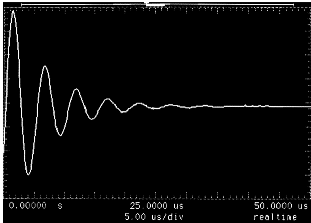
Rys. 33.3. Przebieg na ekranie oscyloskopu pokazujący, że drgania w obwodzie RLC w rzeczywistości znikają, gdyż energia jest rozpraszana na oporniku w postaci energii termicznej
