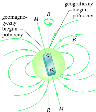
Rys. 32.4. Pole magnetyczne Ziemi przedstawione jako pole dipola. Oś dipola MM tworzy kąt 11,5^\circ z osią obrotu Ziemi RR . Południowy biegun dipola znajduje się na półkuli północnej
