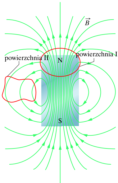
Rys. 32.3. Linie pola magnetycznego krótkiego magnesu sztabkowego. Krzywe zamknięte zaznaczone na czerwono są przekrojami trójwymiarowych powierzchni Gaussa
