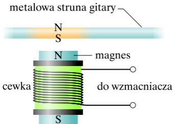
Rys. 31.7. Widok z boku przetwor- nika gitary elektrycznej. Pobudzenie do drgań metalowej struny (która zacho- wuje się jak magnes), powoduje zmianę strumienia magnetycznego, która indu- kuje prąd w cewce
