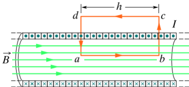
Rys. 30.19. Zastosowanie prawa Amperè'a do odcinka długiego idealnego solenoidu, w którym płynie prąd o natężeniu I . Kontur całkowania jest prostokątem abcd
