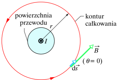
Rys. 30.13. Zastosowanie prawa Amperè'a do wyznaczenia indukcji magnetycznej pola, wytworzonego przez prąd o natężeniu I , płynący w długim prostoliniowym przewodzie. Konturem całkowania jest okrąg, leżący na zewnątrz przewodu
