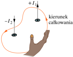
Rys. 30.12. Reguła prawej dłoni dla prawa Ampère'a, służąca do określenia znaków prądów objętych konturem. Sytuacja odpowiada przedstawionej na rysunku 30.11
