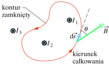
Rys. 30.11. Prawo Ampère'a zastosowane do dowolnego konturu, który obejmuje dwa długie prostoliniowe przewody, ale nie obejmuje trzeciego przewodu. Zwróć uwagę na kierunki prądów
