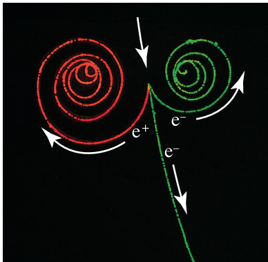
Rys. 29.2. Ślady dwóch elektronów ( e^- ) i pozytonu ( e^+ ) w komorze pęcherzykowej, umieszczonej w jednorodnym polu magnetycznym, które jest skierowane prostopadle przed płaszczyzną rysunku
