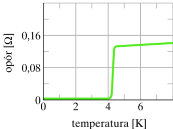
Rys. 27.13. Opór rtęci maleje do zera przy temperaturze około 4 K
