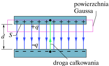
Rys. 26.4. Naładowany kondensator płaski. Powierzchnia Gaussa obejmuje ładunek na okładce dodatniej. Całkowanie we wzorze (26.6) wykonujemy wzdłuż odcinka, od okładki ujemnej do okładki dodatniej
