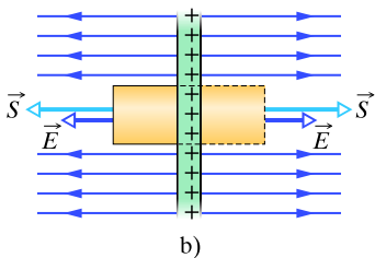
Rys. 24.15. Widok a) z ukosa, b) z boku fragmentu bardzo dużej, cienkiej płyty plastikowej, naładowanej jednorodnie z jednej strony z gęstością powierzchniową ładunku \sigma . Zamknięta walcowa powierzchnia Gaussa przenika przez płytę i jest prostopadła do niej
