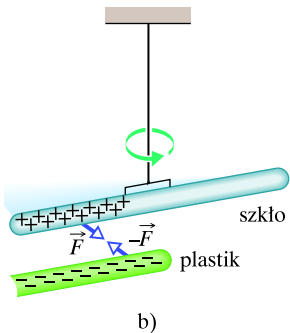
Rys. 22.1. a) Dwa pręty naładowane ładunkami tego samego znaku się odpychają. b) Dwa pręty naładowane ładunkami o przeciwnych znakach się przyciągają. Znaki plus oznaczają wypadkowy ładunek dodatni, a znaki minus — wypadkowy ładunek ujemny
