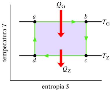
Rys. 21.9. Cykl Carnota z rysunku 21.8 przedstawiony we współrzędnych temperatura-entropia. W przemianach ab i cd temperatura jest stała. W przemianach bc i da entropia jest stała
