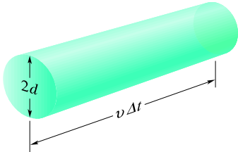
Rys. 20.6. W czasie \Delta t poruszająca się cząsteczka „przemiała” walec o wysokości v\Delta t i promieniu d
