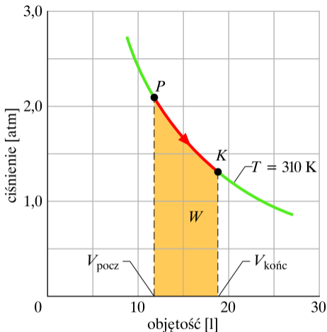
Rys. 20.2. Przykład 20.2. Zacięziony obszar odpowiada pracy wykonywanej przez 1 mol tlenu, który w stałej temperaturze T równej 310 K rozszerza się od objętości V_{\text{pocz}} do V_{\text{końc}}
