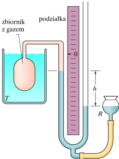
Rys. 19.5. Termometr gazowy o stałej objętości. Zbiornik zanurzono w cieczy, której temperatura T jest mierzona
