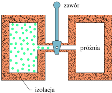
Rys. 19.16. Otwarcie zaworu między dwiema komorami powoduje swobodne rozprężenie gazu. Gaz wypełnia obydwie komory i w końcu osiąga stan równowagi
