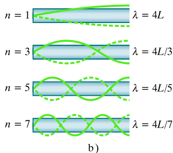
Rys. 18.13. Fale stojące w strunie narysowane na tle rur przedstawiają stojące fale dźwiękowe w rurach. a) Gdy oba końce rury są otwarte, możliwe jest wzbudzenie każdej harmonicznej (patrz także rysunek 18.12). b) Gdy otwarty jest jedynie jeden koniec rury, wzbudzić można jedynie nieparzyste harmoniczne
