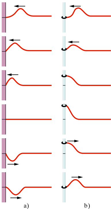
Rys. 17.19. a) Impuls padający z prawej strony odbija się od lewego końca liny umocowanej do ściany. Zauważmy, że impuls odbity jest odwrócony względem impulsu padającego. b) Na tym rysunku lewy koniec liny jest umocowany do pierścienia, który może się ślizgać bez tarcia w górę i w dół wzdłuż pręta. W tym przypadku impuls nie ulega odwróceniu przy odbiciu
