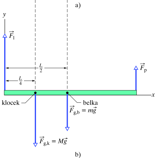
Rys. 13.5. Przykład 13.1. a) Belka o masie m podtrzymuje klocek o masie M . b) Diagram sił działających na układ belka + klocek
