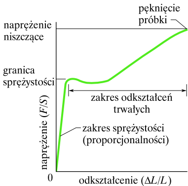
Rys. 13.13. Zależność odkształcenia od naprężenia dla próbki ze stali o kształcie jak na rysunku 13.12. Próbkę ulega odkształceniu trwałemu po przekroczeniu przez naprężenie granicy sprężystości materiału. Próbkę pęka po osiągnięciu przez naprężenie wartości odpowiadającej naprężeniu niszczącemu dla badanego materiału
