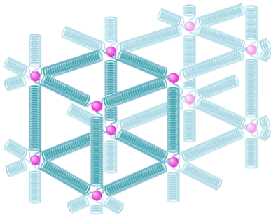
Rys. 13.10. Atomy metalicznego ciała stałego są regularnie ułożone w trójwymiarowej sieci. Sprężynki symbolizują siły działające między atomami
