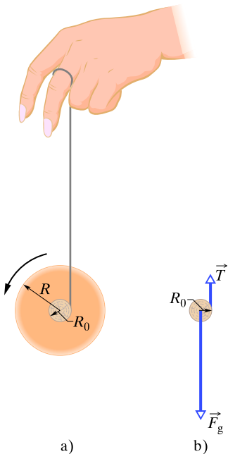
Rys. 12.8. a) Przekrój zabawki jo-jo. Wokół osi o promieniu R_0 nawinięty jest sznurek, którego grubość pomijamy. b) Diagram sił działających na opadające kółko (pokazano tylko jego ośkę)
