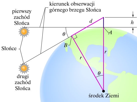
Rys. 1.3. Przykład 1.4. Linia, wzdłuż której patrzysz na zniknięcie Słońca za horyzontem obraca się o kąt \theta gdy wstajesz, a więc podnosisz oczy na wysokość h nad punkt A (dla wyrazistości rysunku kąt \theta i odcinek h narysowano przesadnie duże)
