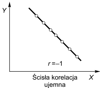
Rysunek 19.5. Wartości współczynnika korelacji
