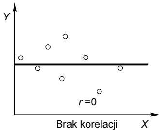
Rysunek 19.5. Wartości współczynnika korelacji
