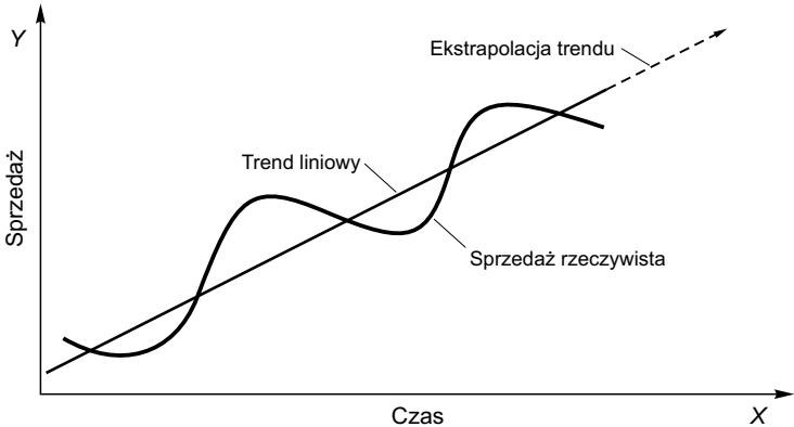
Rysunek 19.3. Model linii prostej trendu i ekstrapolacja trendu
